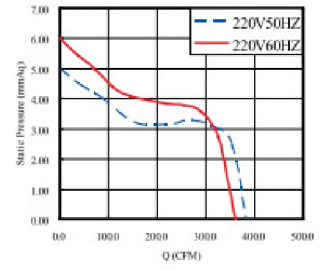
CA06060V22F
